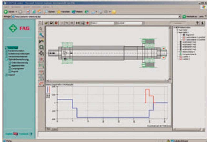
42: Cálculo de la distribución de la carga de un husillo
